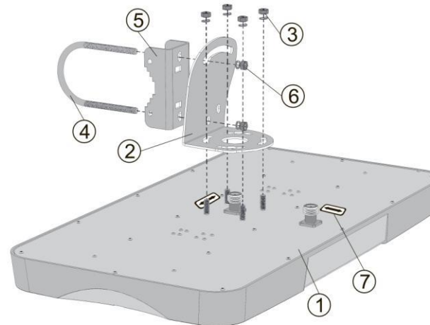
Рис. 2 Сборка антенны
