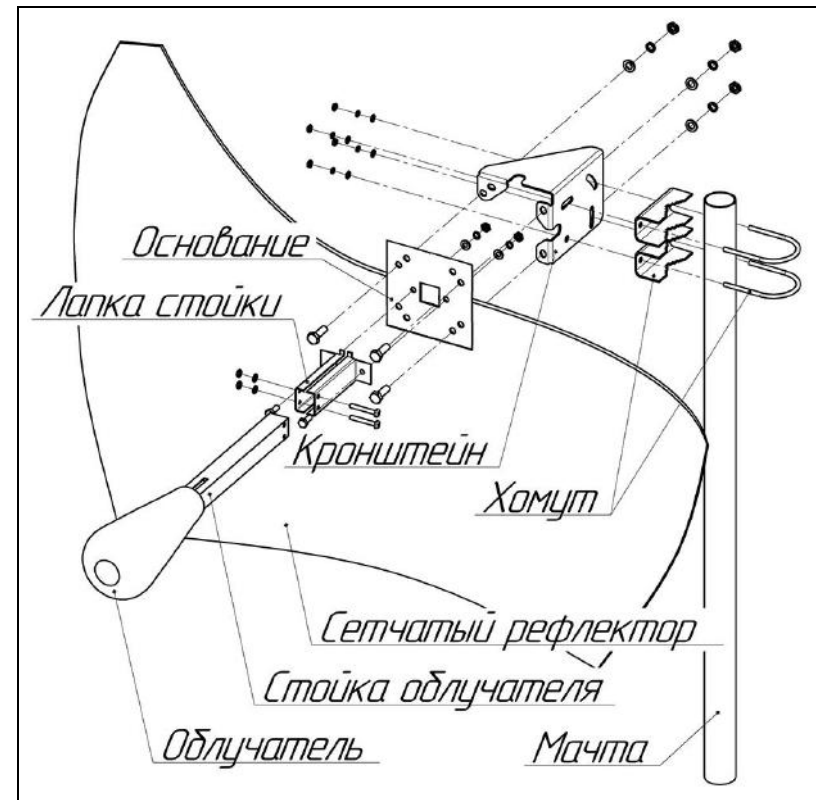
Схема 1 – Сборка антенны
