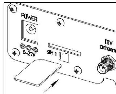
Рисунок 1- Установка SIM-карты
